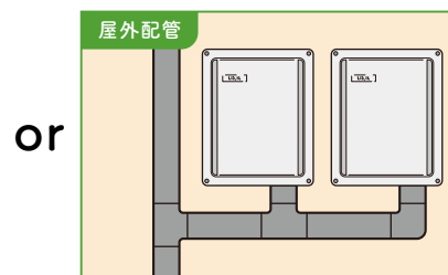
屋外配管 パワーコンディショナへの配管・配線が 外壁材の外側を通ります。
